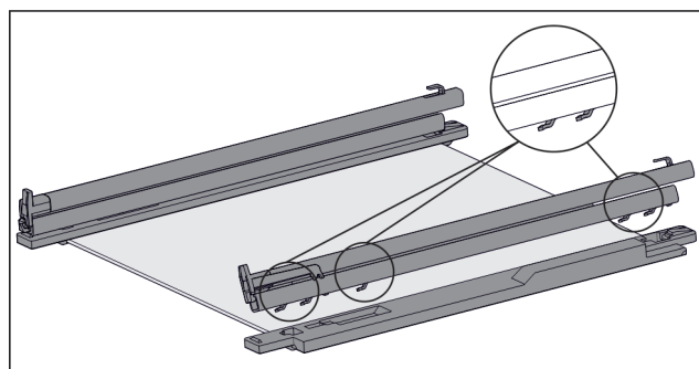
Fig. 44 Skleněná deska s kolejničkami a přídržnými díly
